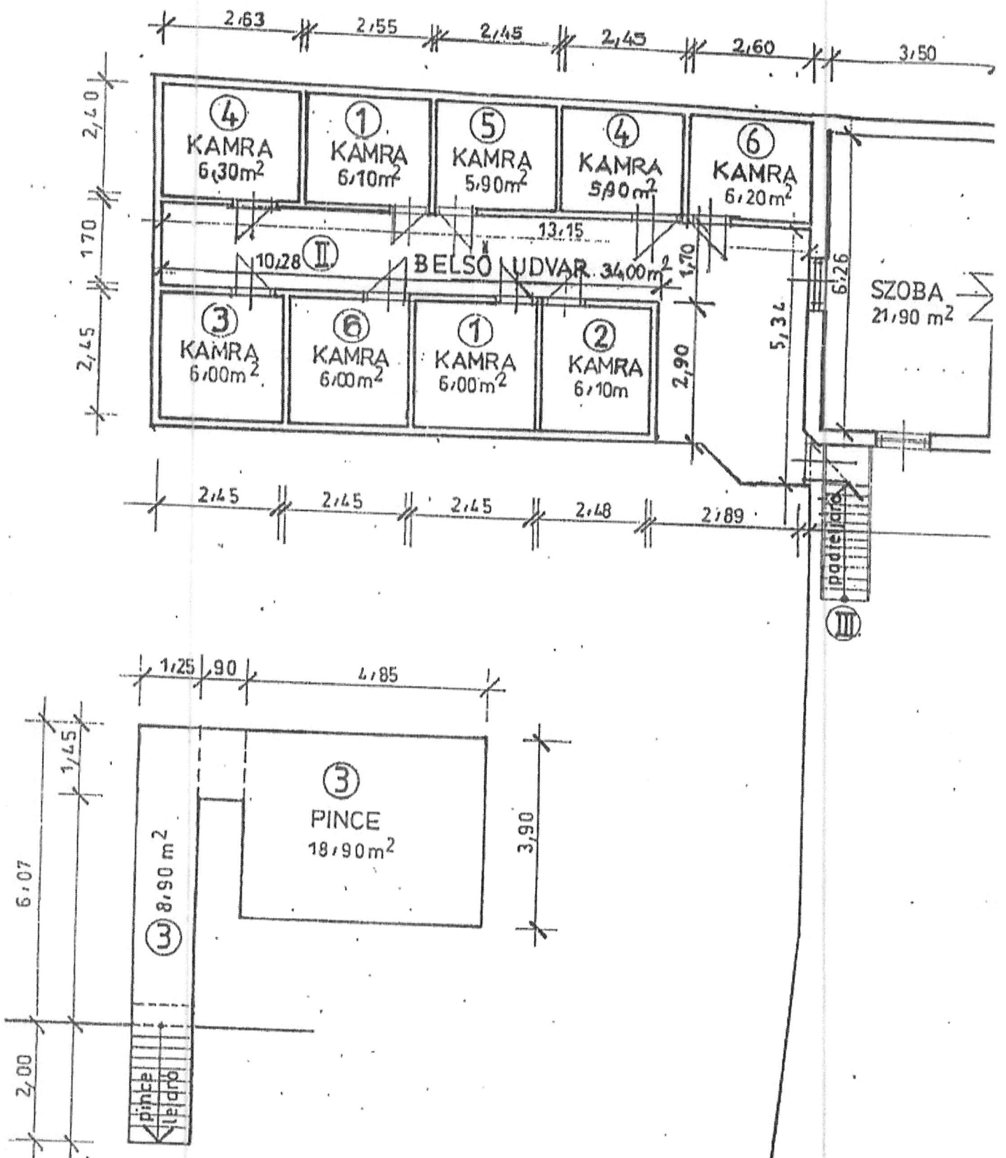
PINCÉ ALAPRAJZ M=1:100
