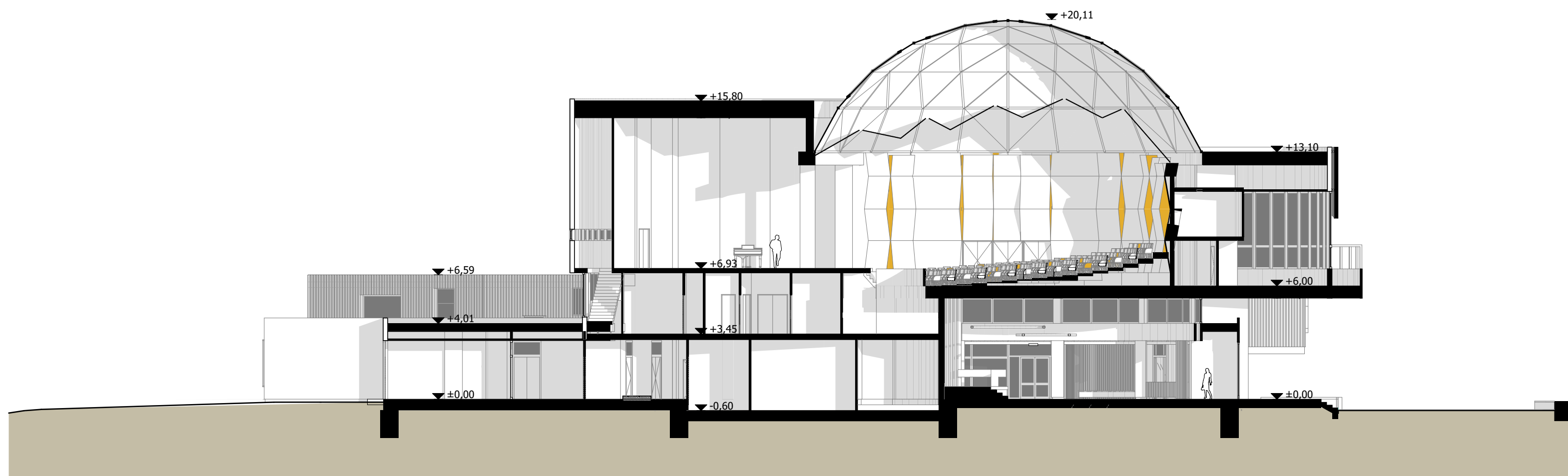
A-A METSZET
