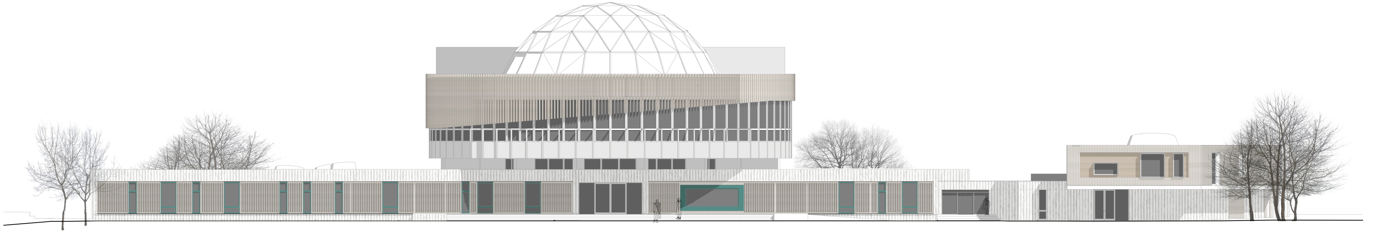
ÉSZAKKELETI HOMLOKZAT
