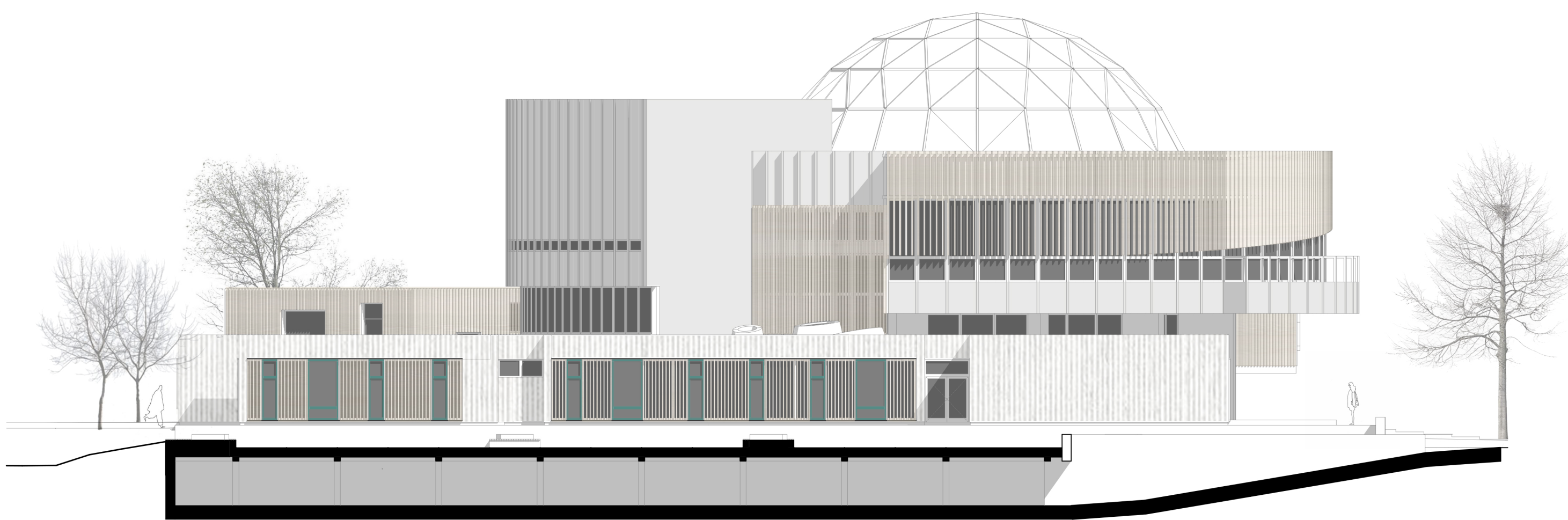
DÉLKELETI HOMLOKZAT
