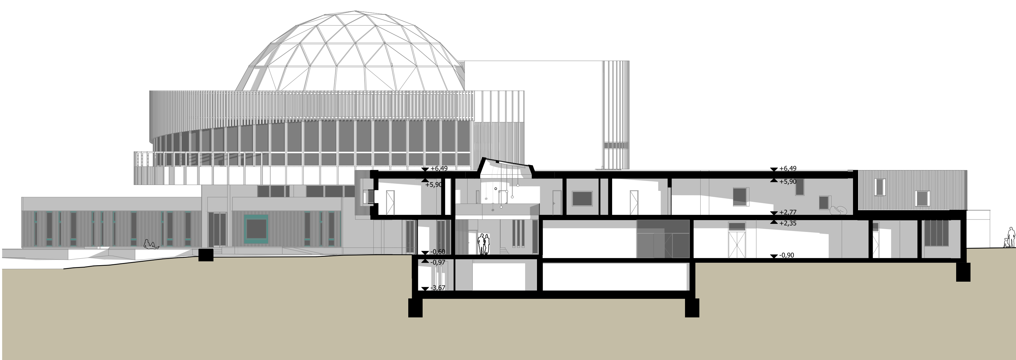
B-B METSZET
